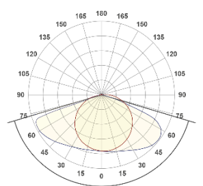
Işık Şiddeti Dağılım Eğrisi Light Intensity Distribution Curve
