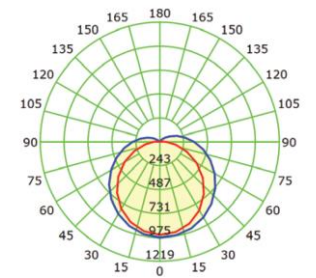
Işık Şiddeti Dağılım Eğrisi Light Intensity Distribution Curve
